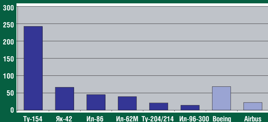
Основные типы магистральных пассажирских самолетов в парке гражданской авиации России в 2005 г.
