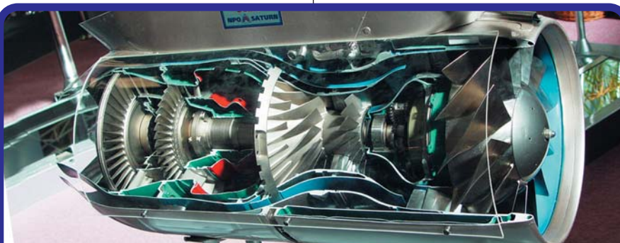
Современные малоразмерные короткоресурсные двигатели для БПЛА имеют конструкцию с малым числом деталей. Не снимке – ТРДД типа 36МТ в разрезе
